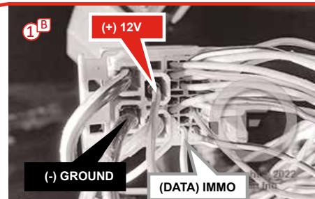
X4 Gray connector Connecteur Gris X4
